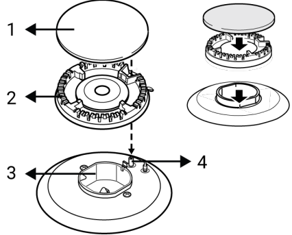
1 غطاء الشعلة
