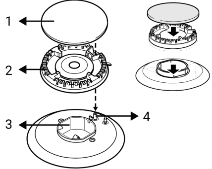
غطاء الشعلة
